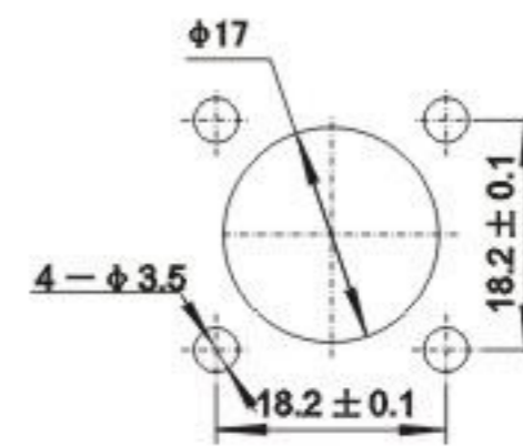
安装开孔尺寸 Mounting hole
